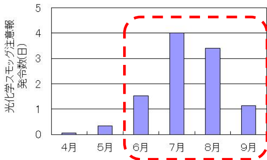
神奈川県内における光化学スモッグ注意報 月別発令状況 (平成12～平成26年平均値)
